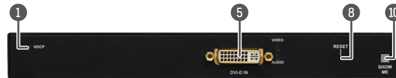
DVI-HDCP-TPS-TX220
